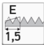
ŘEZNÝ KUŽEL E Délka 1,5 stoupání
