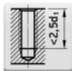
TYP OTVORU Neprůchozí (délka závitu L < 2,5 \times d1 )
